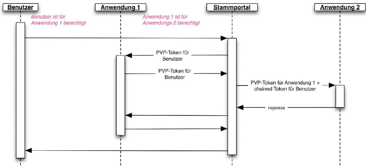
Abbildung 1: Beispiel zu Chained-Token
